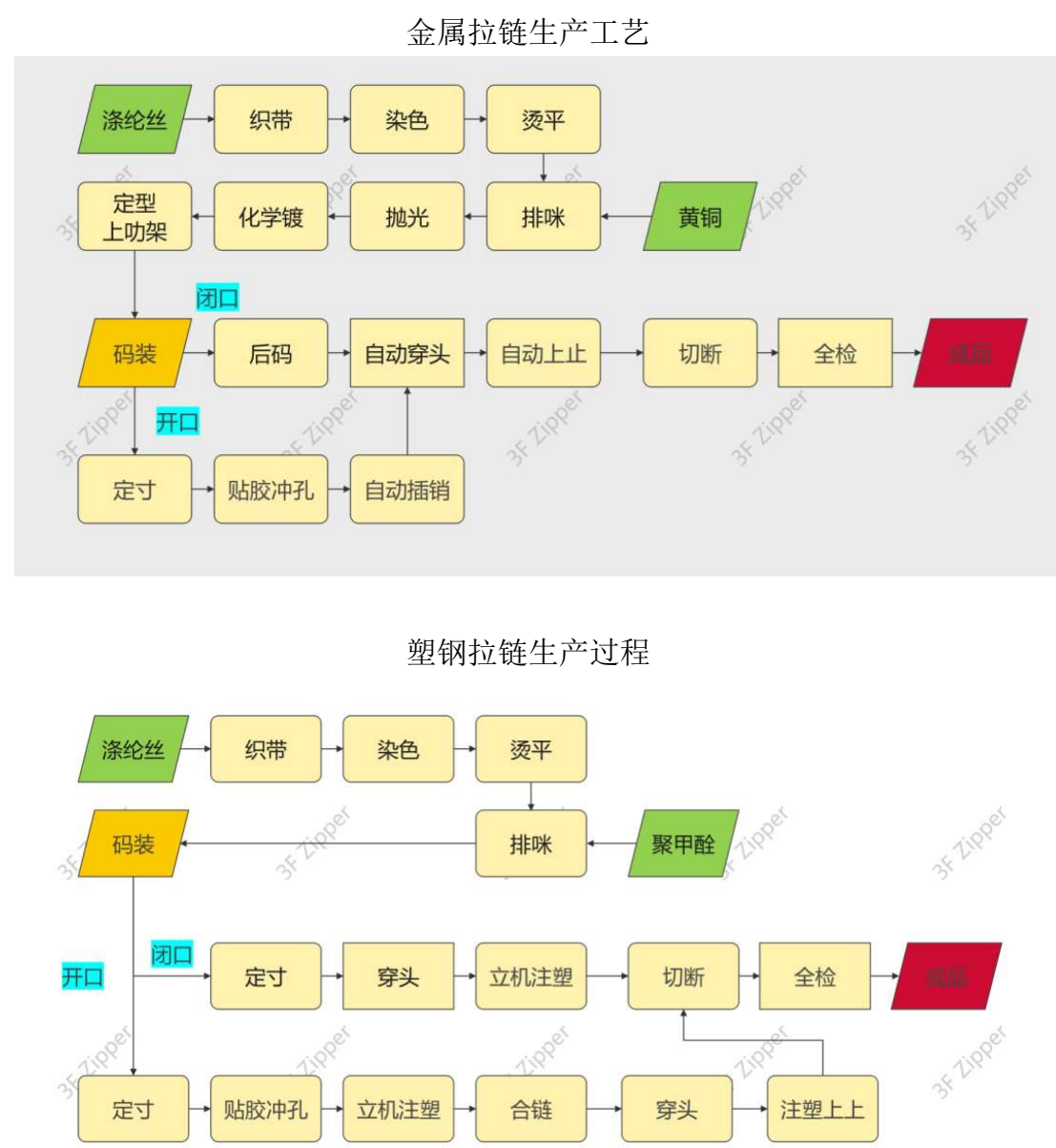
图 3-1 受核查方生产工艺流程图
